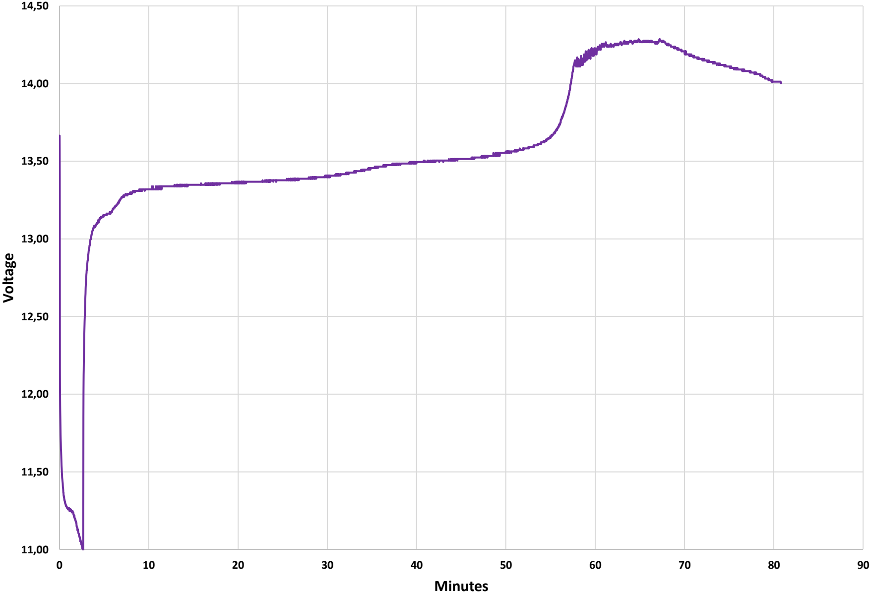
Cycle décharge @ 90 ampères - charge @ 5 ampères
